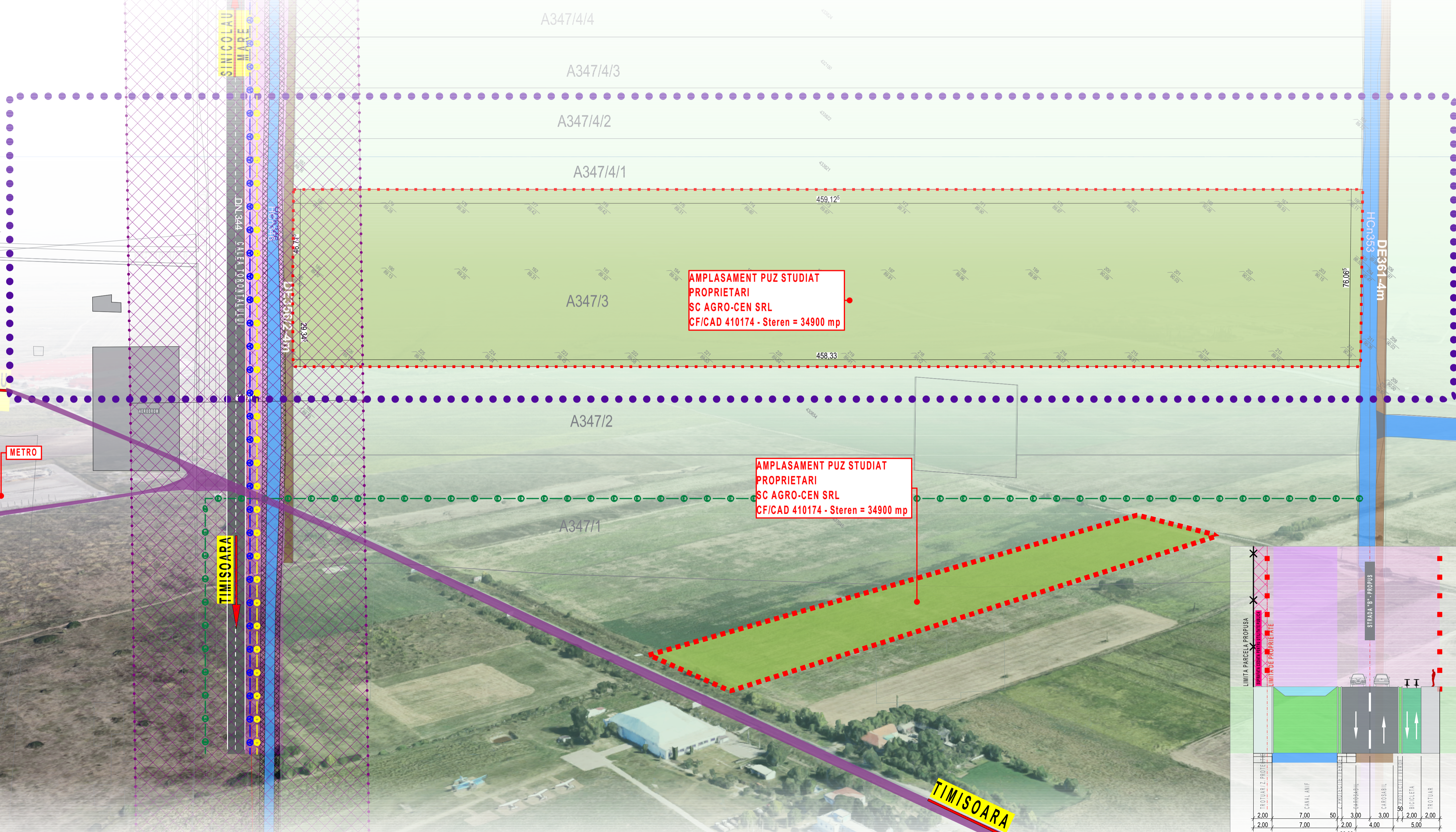
PLAN DE SITUATIE - EXISTENT 1:1000
