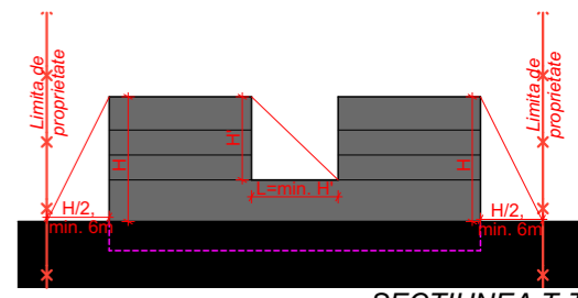
SECTIUNEA T-T
