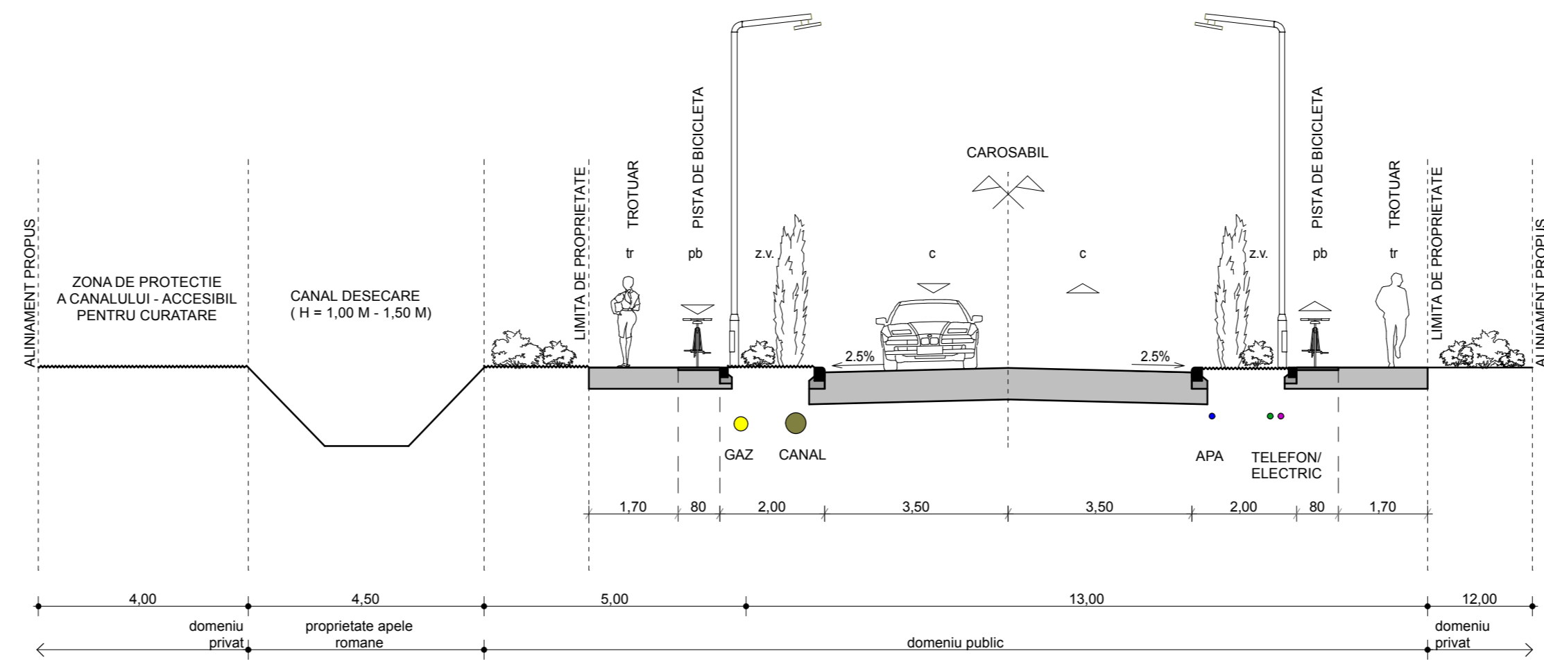
PROFIL TRANSVERSAL TIP 1b - 16m STRADA PRINCIPALA (2 benzi) SI CANAL ADIACENT
