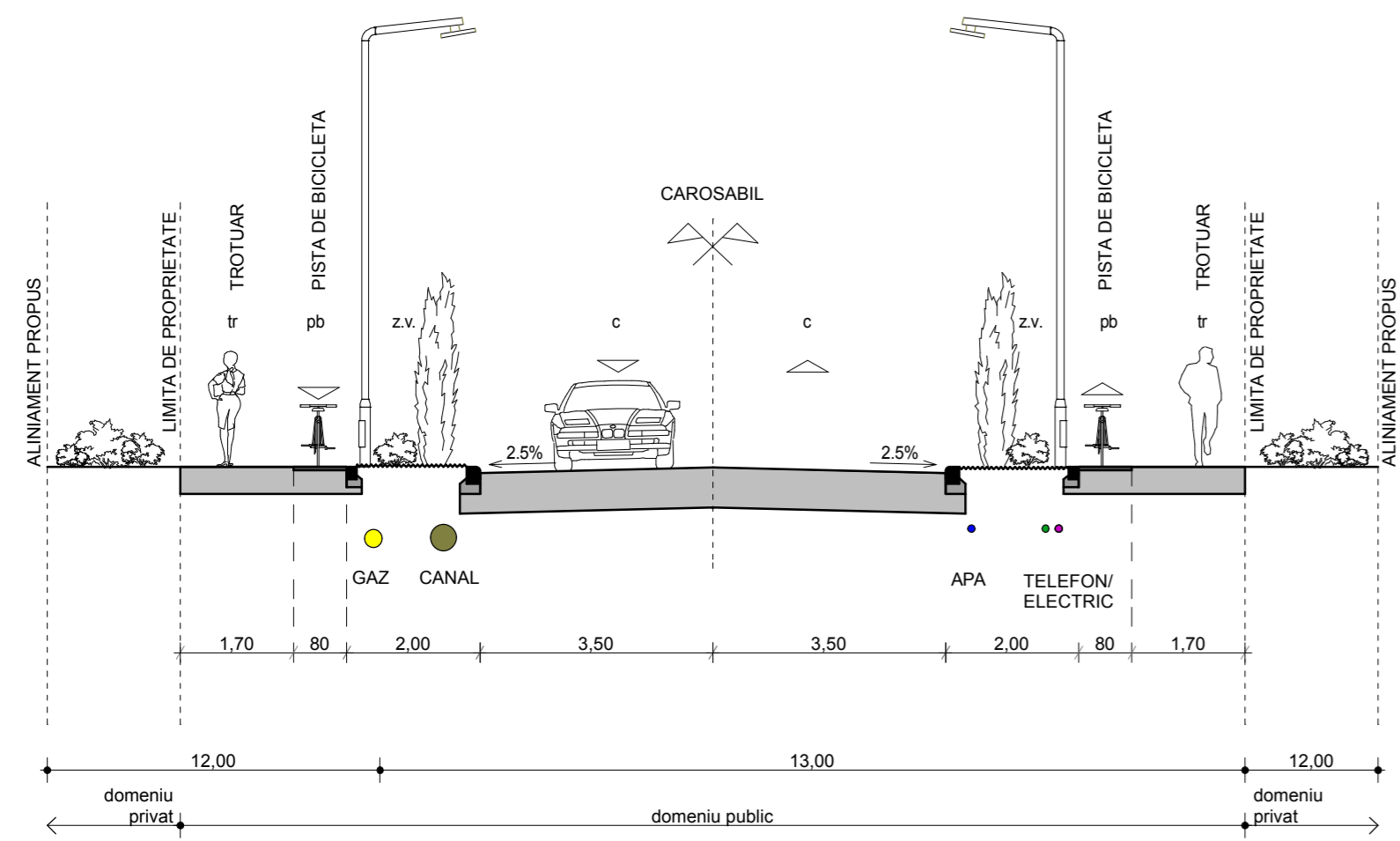
PROFIL TRANSVERSAL TIP 1a - 16m STRADA PRINCIPALA (2 benzi) SI CANAL ADIACENT
