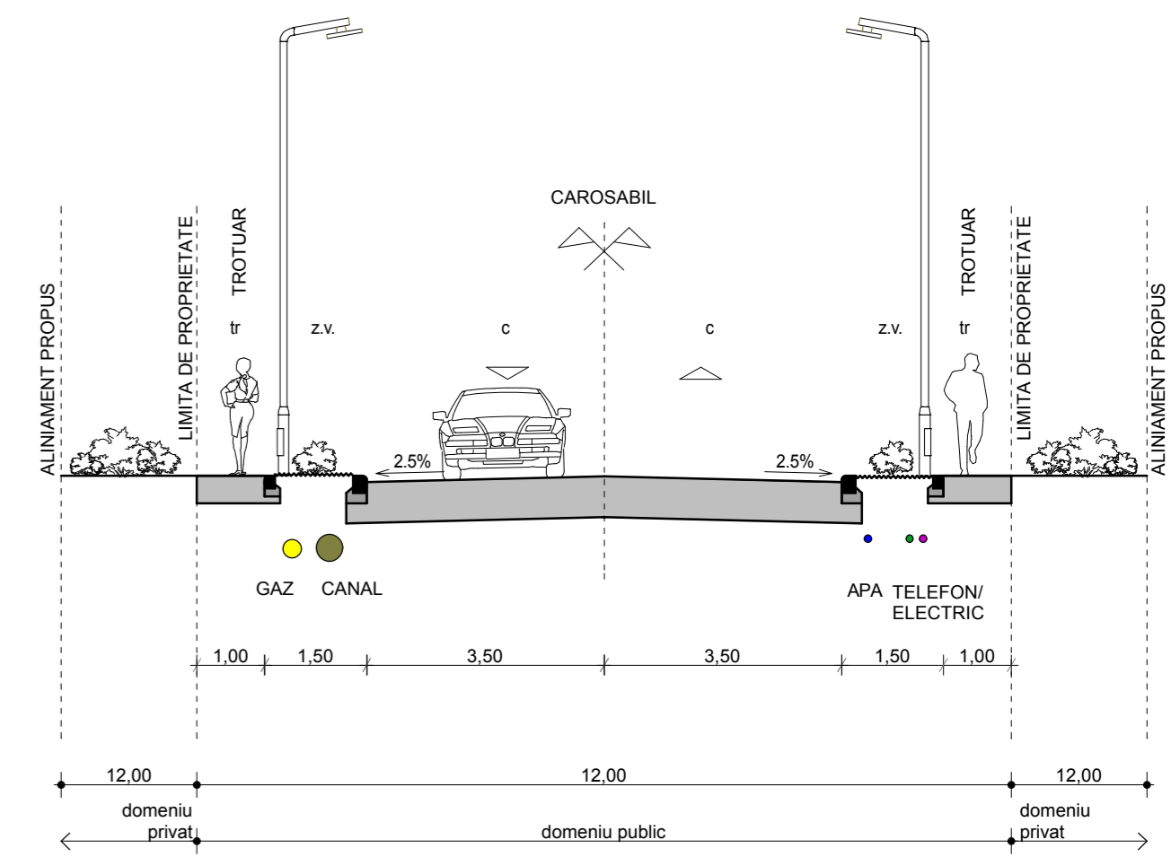
PROFIL TRANSVERSAL TIP 2a - 12m STRADA SECUNDARA (2 benzi)
