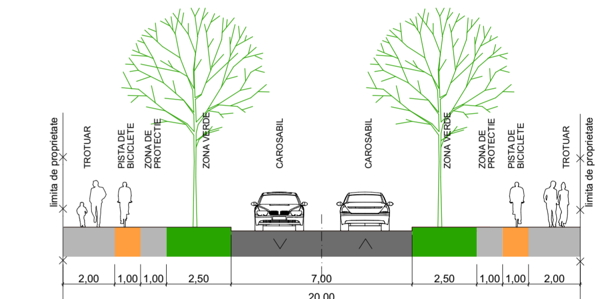
PROFIL STRADAL PTT16 (20m) PROPUZ PRIN NOUL PUG (ETAPA3, REVIZIA 3, ANEXA 6) / CONSTITUIT PARTIAL PRIN PUZ APROBAT PRIN HCL 69/2014 (nr. cad. 436113) SI PRIN PUZ CONFORM A.O. NR. 26/14.07.2017 (nr.cad. 442196)
