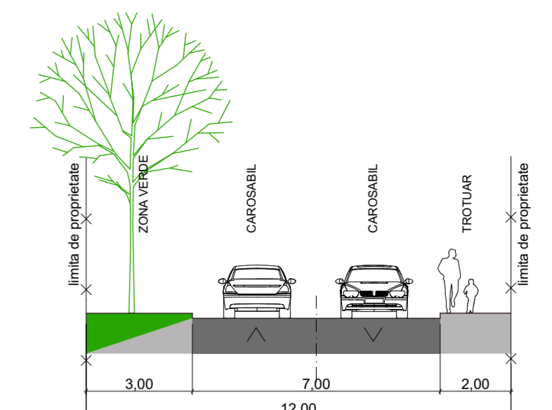
PROFIL STRADAL PTT2 (12m) DE 1553 REGLEMENTAT PRIN PUD APROBAT PRIN HCL 334/2005 SI PUZ APROBAT PRIN HCL 75/2010 (INCLUSIV LEGATURA CU STR. OLARILOR)
