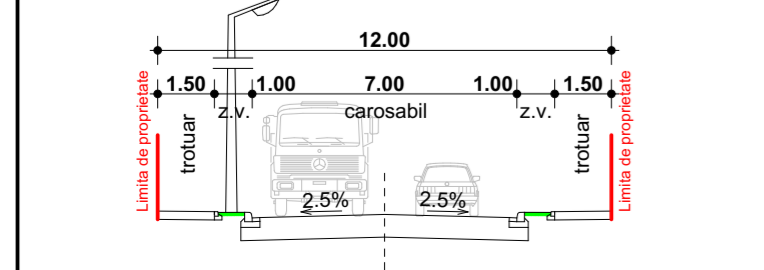
PROFIL TRANSVERSAL PROPUȘ PTT1
