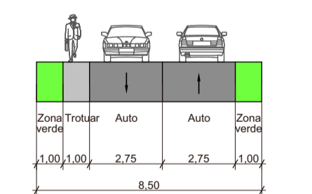
Profil Transversal - 8,5 m Drum de incintă
