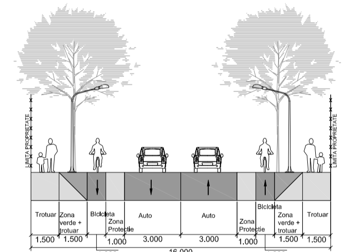
Profil Transversal 67 - lățime 16m
