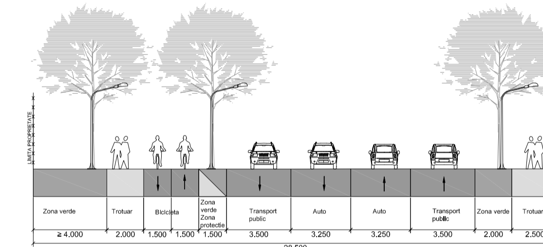
Profil Transversal 52 - lățime 28.5m
