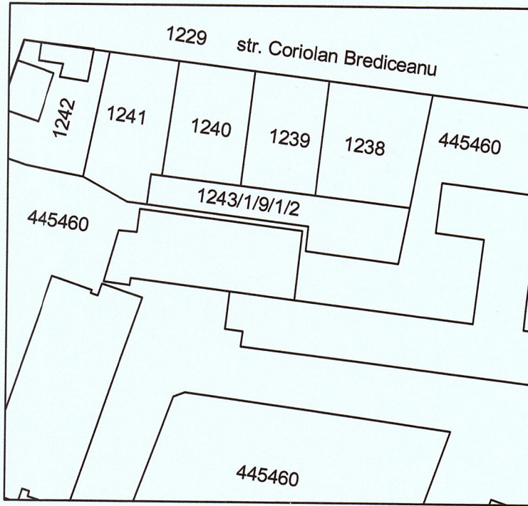
PLAN PARCELAR CONFORM CF SCARA 1:1000
