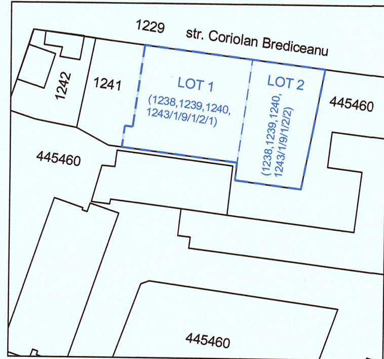
PLAN PARCELAR DUPA DEZLIPIRE SCARA 1:1000
