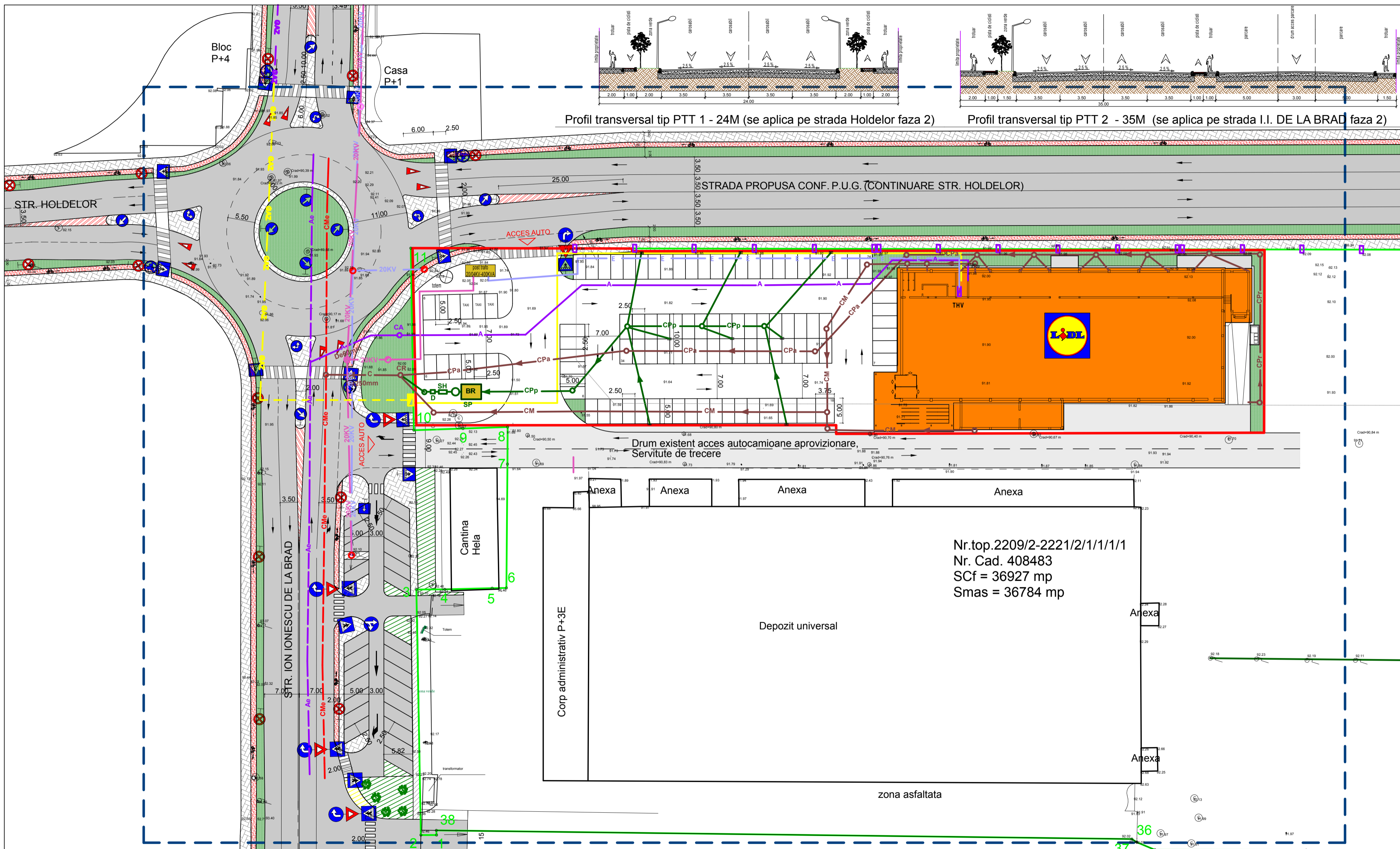
04 REGLEMENTARI - ECHIPARE EDILITARA 1:500
