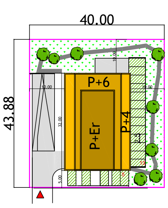
PLAN PARCELA tip B locuinte scara 1:500
