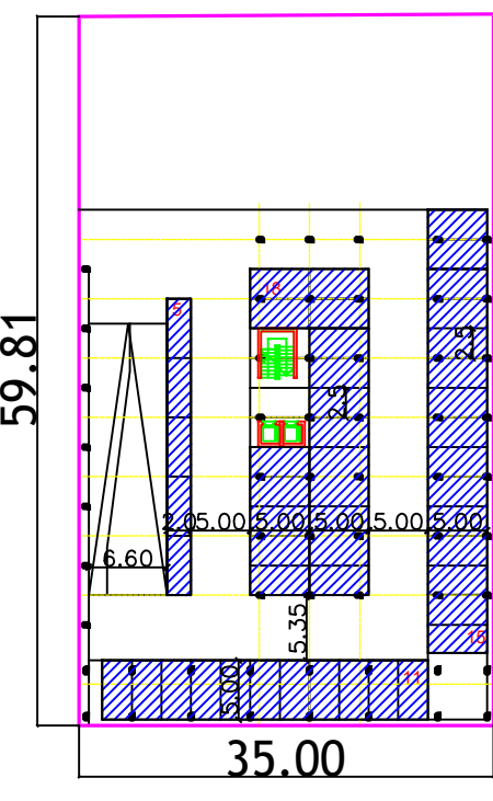
PLAN SUBSOL Parcela tip A scara 1:500
