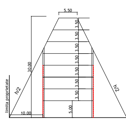
Parcela tip A scara 1:500
