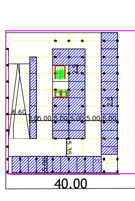
PLAN SUBSOL Parcela tip B scara 1:500
