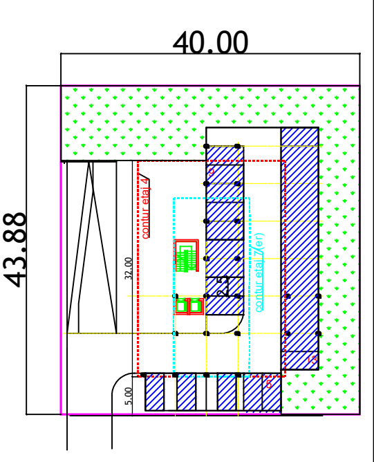
PLAN PARTER Parcela tip B scara 1:500
