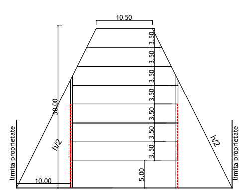
Parcela tip A scara 1:500
