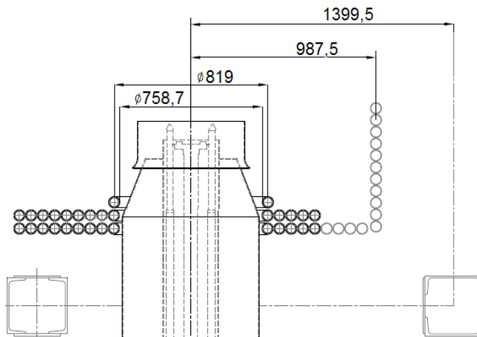
Fig.2.b.1.4.8 Poziționarea noilor arzătoarelor pe perete. Realizarea ambrazurilor
