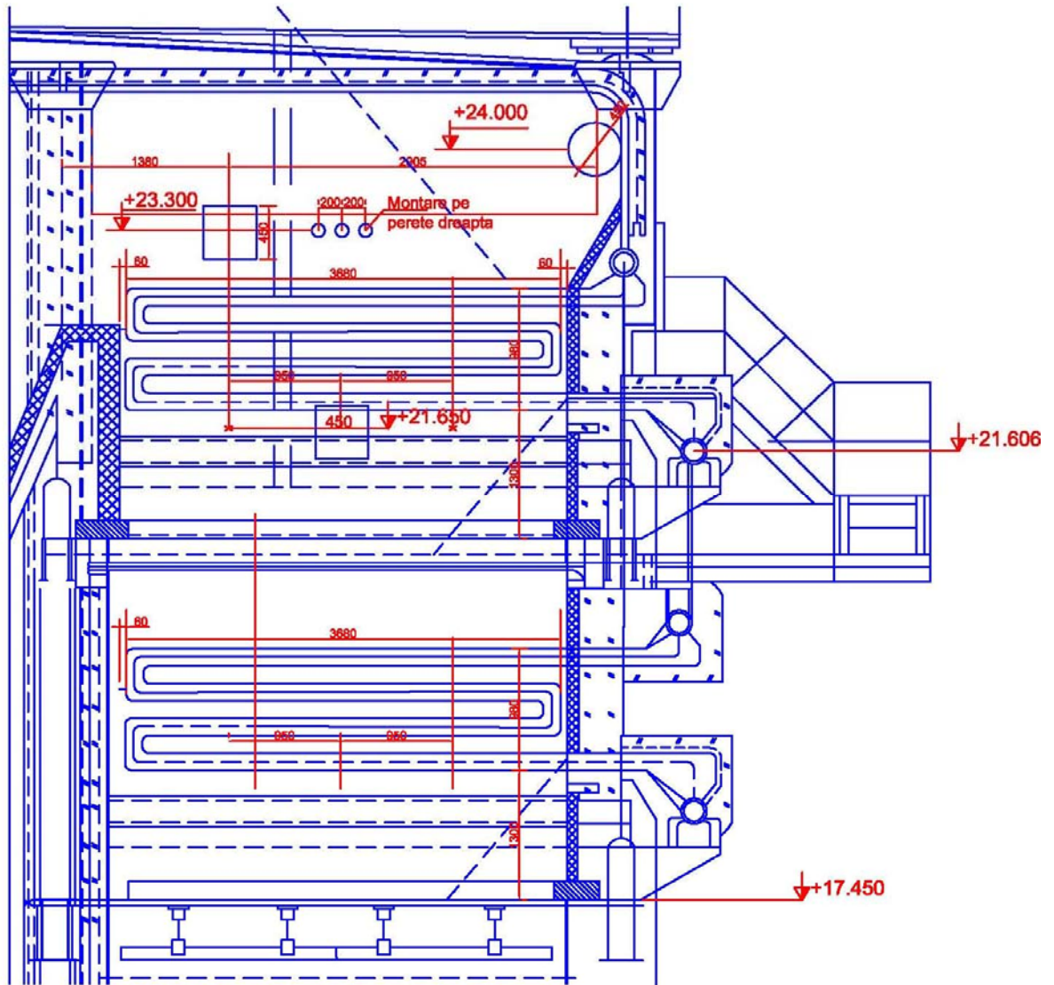
Fig.2.b.1.1.18 Zona supraîncălzitor a cazanului
