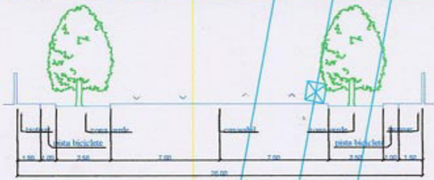
PROFIL STRADAL A-A
