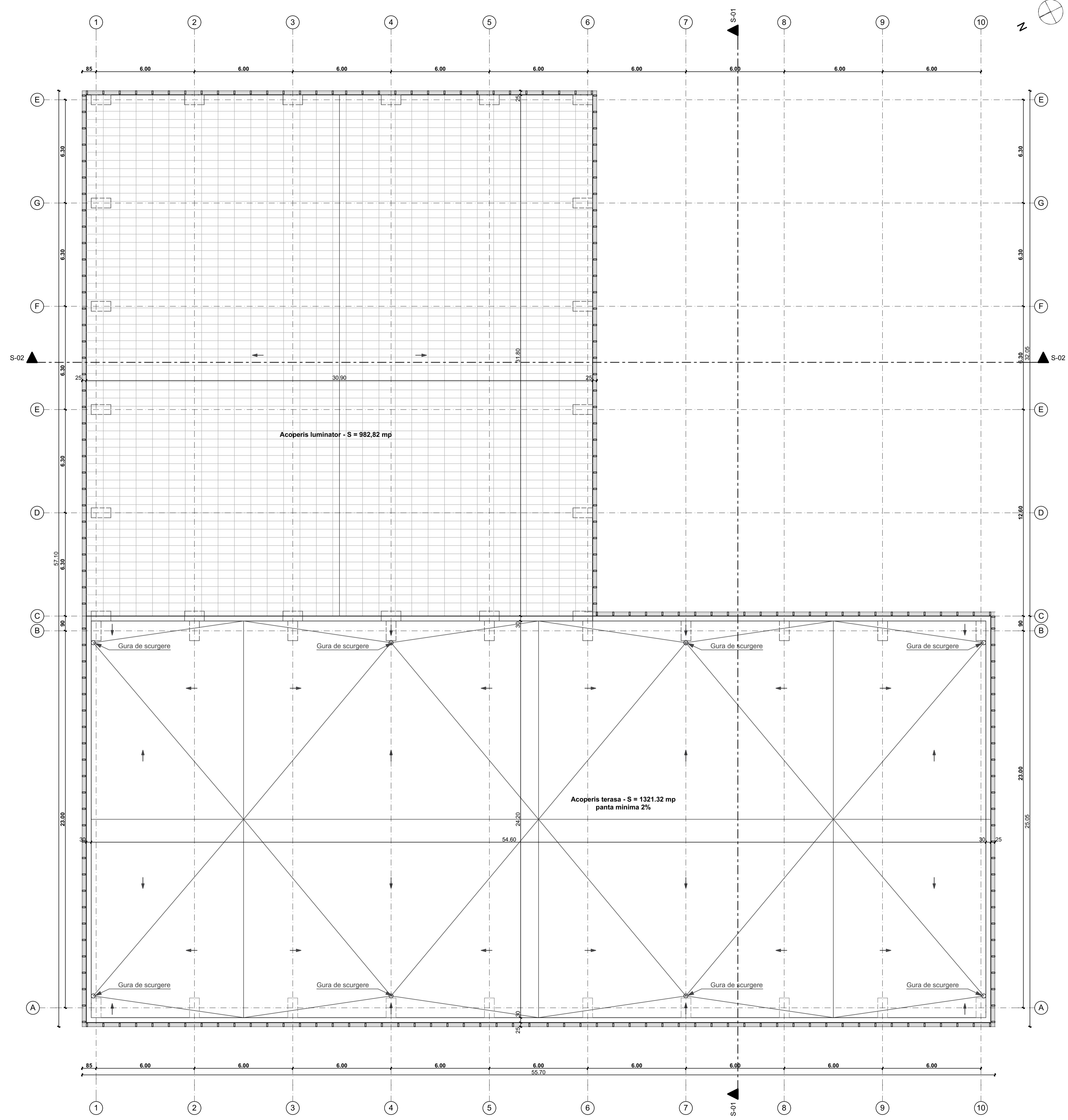
PLAN INVELITOARE - SCARA 1:125
