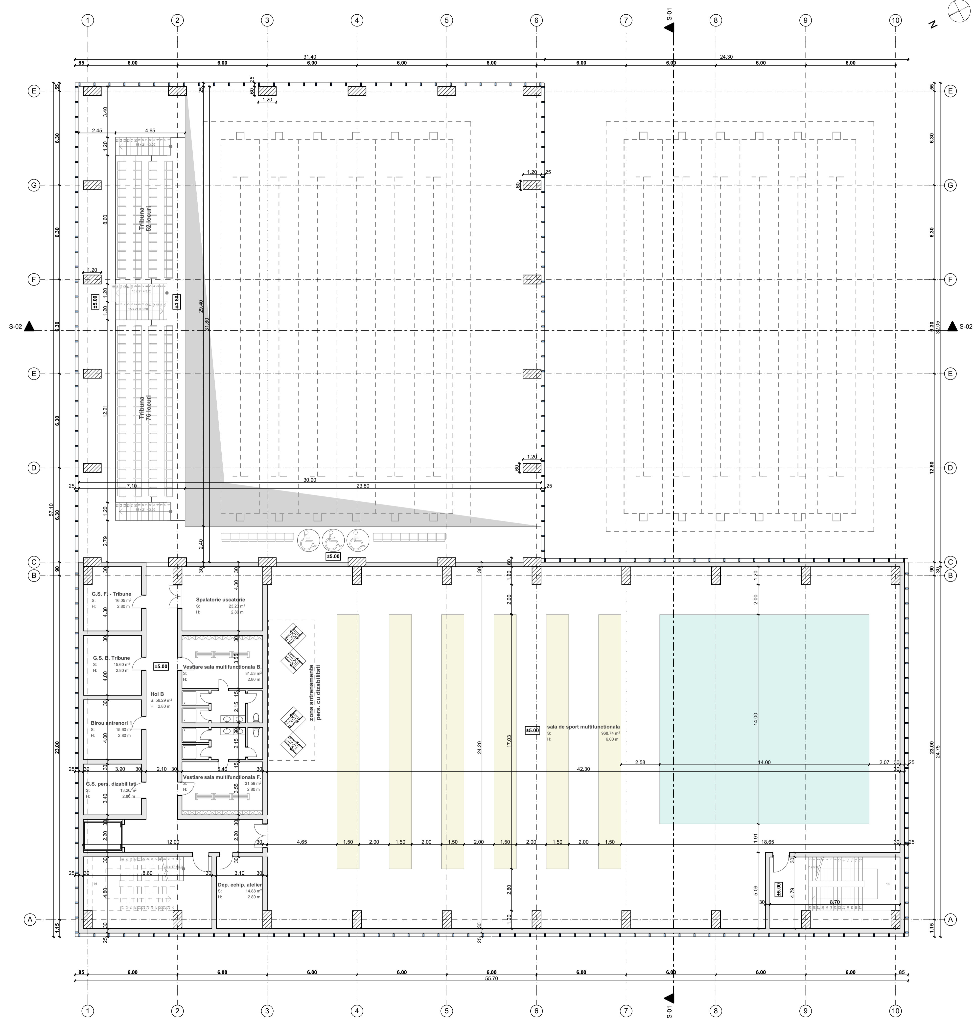
PLAN ETAJ 1 - SCARA 1:125
