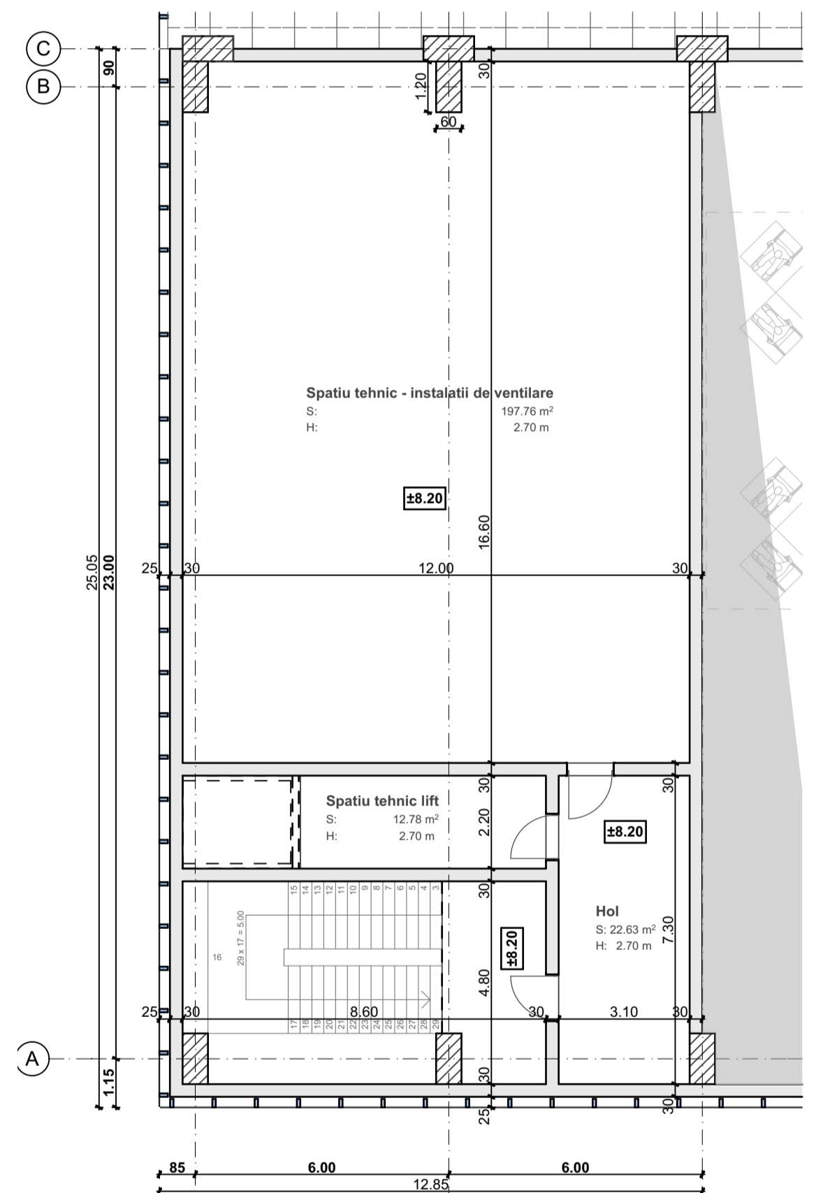
PLAN ETAJ 2 - SCARA 1:125
