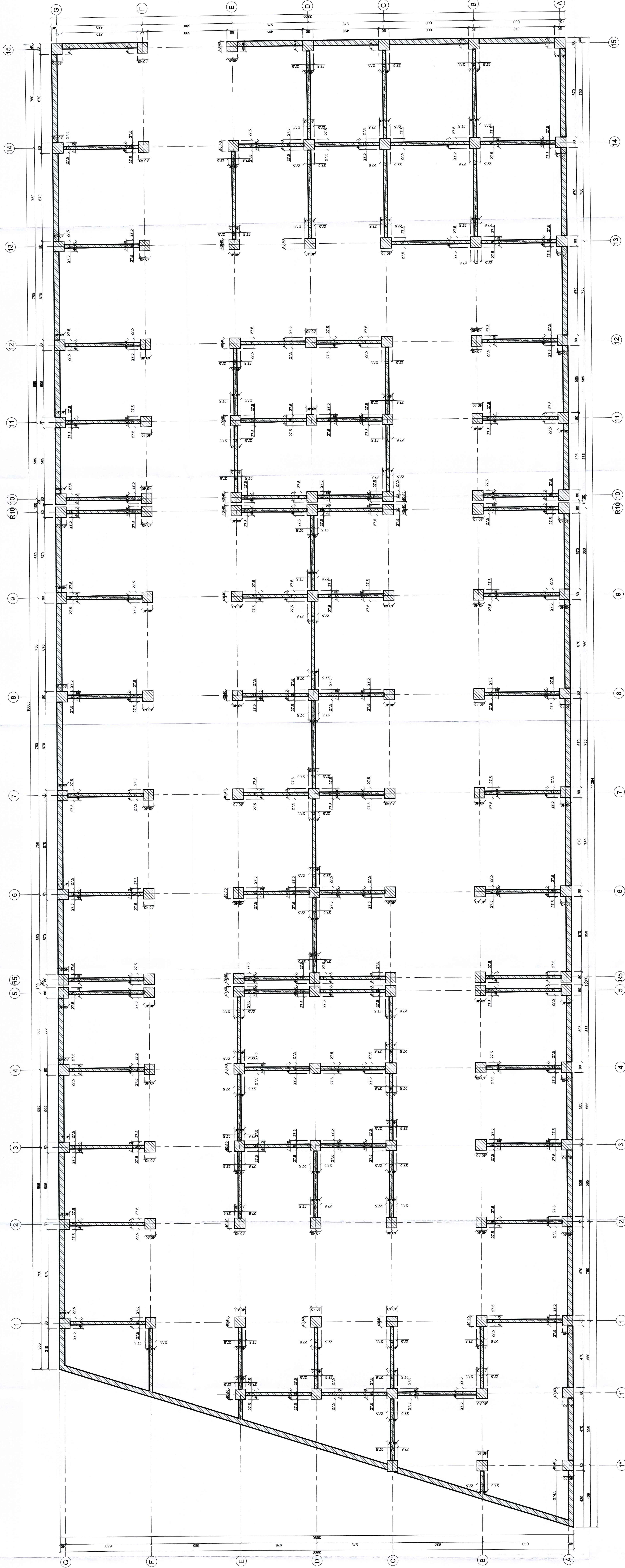
Plan structura de rezistenta subsol Sc. 1:100
