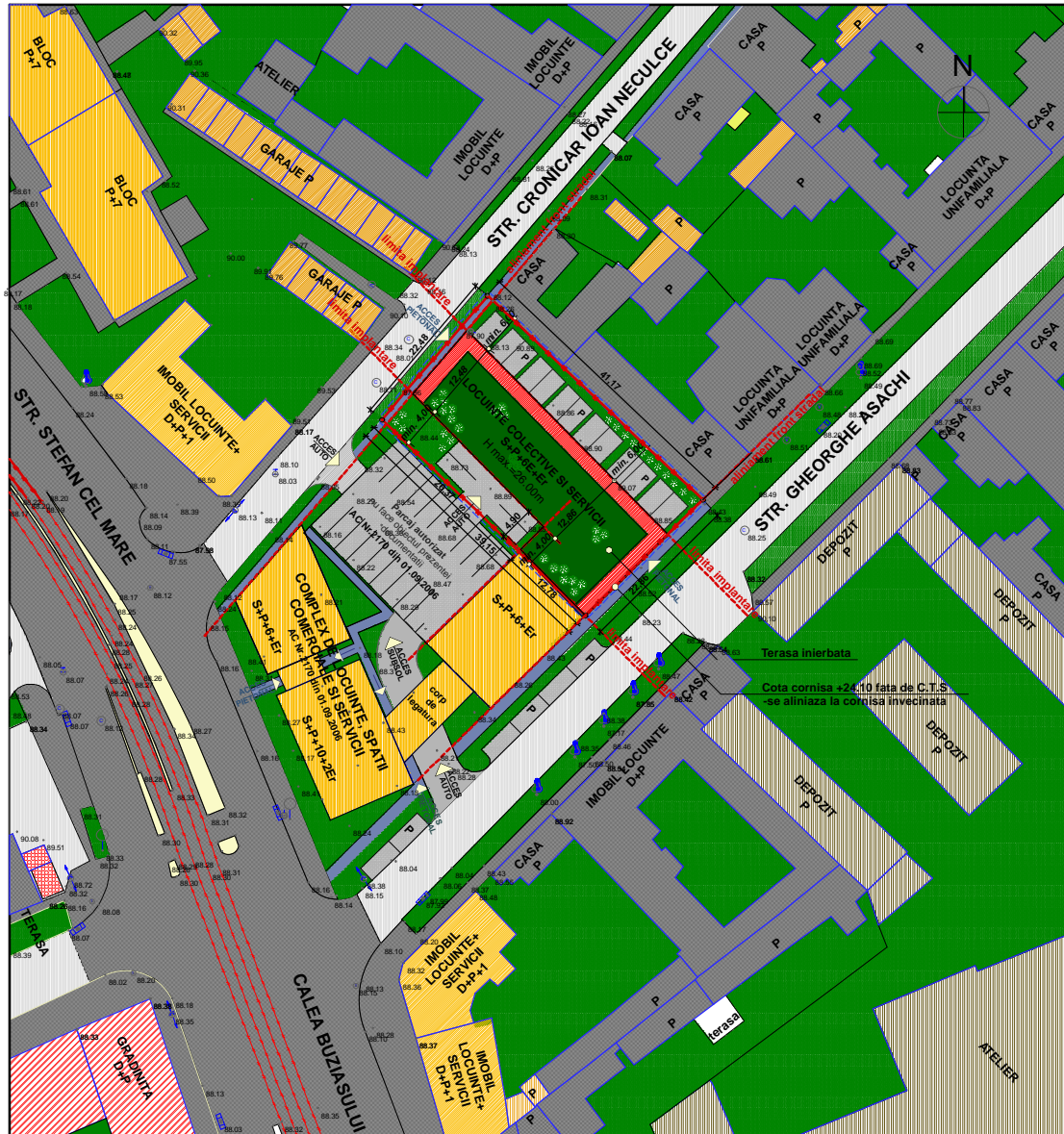
PLAN DE SITUATIE PROPOS SC:1/500
