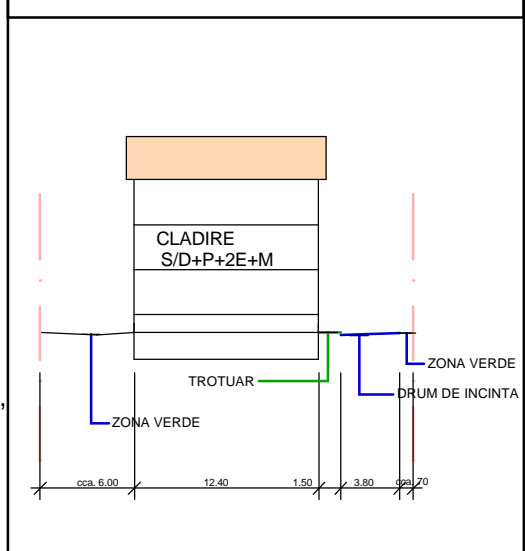
PROFIL STRADAL INCINTA Sc. 1:500
