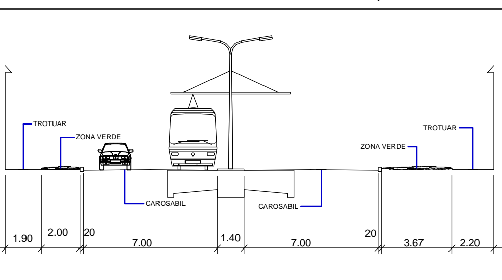
PROFIL STRADAL PROPOS PENTRU STR. I. SLAVICI, Sc. 1:200
