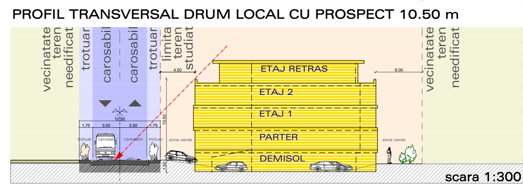
PROFIL TRANSVERSAL DRUM LOCAL CU PROSPECT 10.50 m
