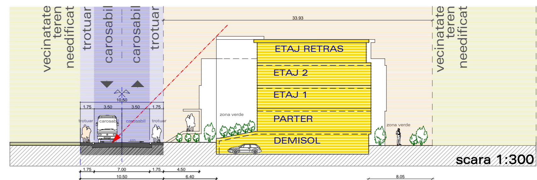
PROFIL TRANSVERSAL DRUM LOCAL CU PROSPECT 10.50 m
