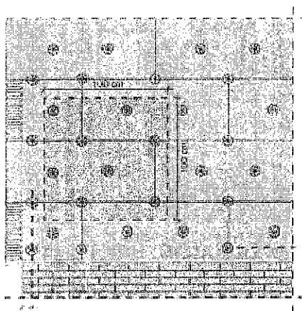
Dispunerea diblurilor pentru fixarea plăcilor din vată minerală bazaltică (MW) în zona colțului, la colț și în câmp curant.
