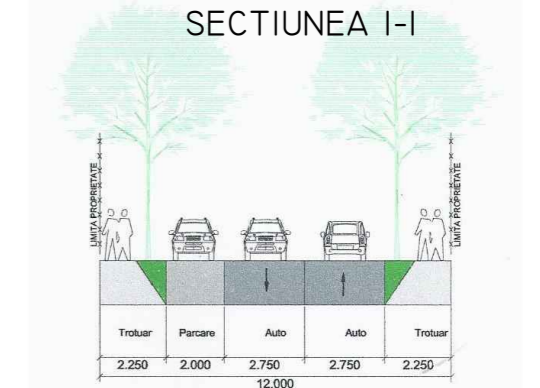
PROFIL TRANSVERSAL DE 12,00M SECTIUNEA 1-1
