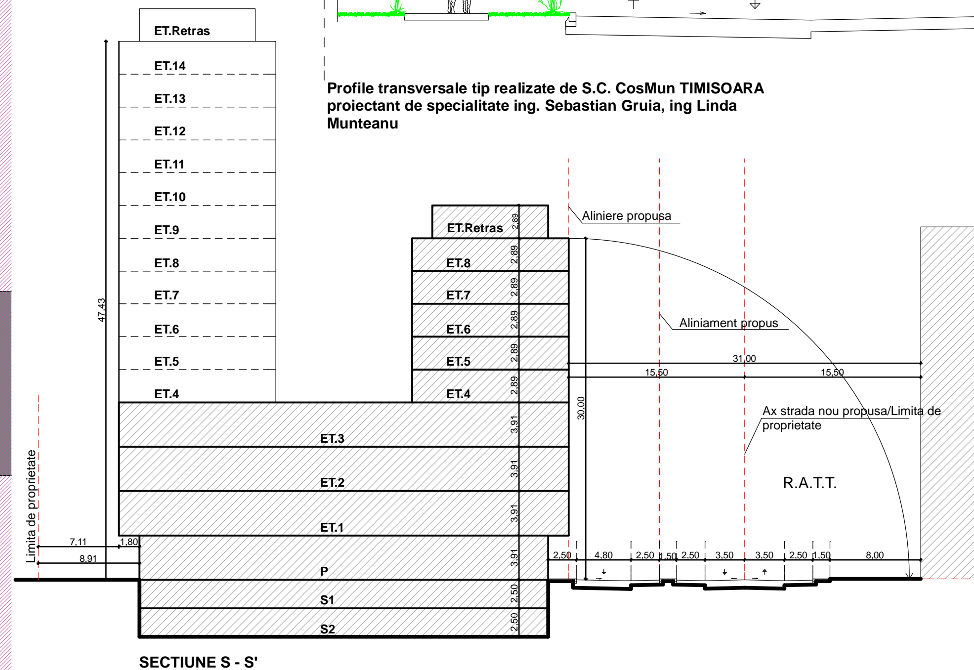
SECTIUNE S - S'
