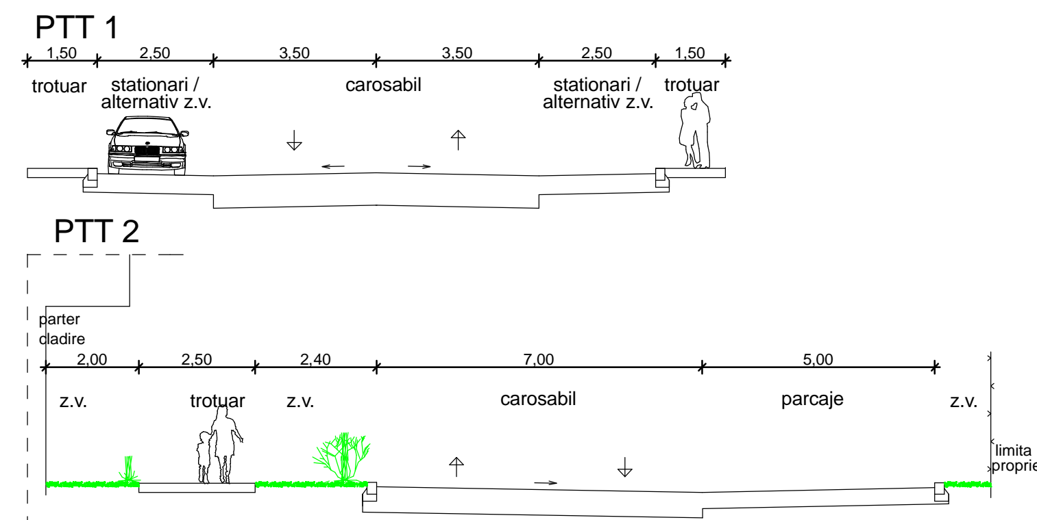
Profile transversale tip realizate de S.C. CosMun TIMISOARA proiectant de specialitate ing. Sebastian Gruiu, ing. Linda Munteanu
