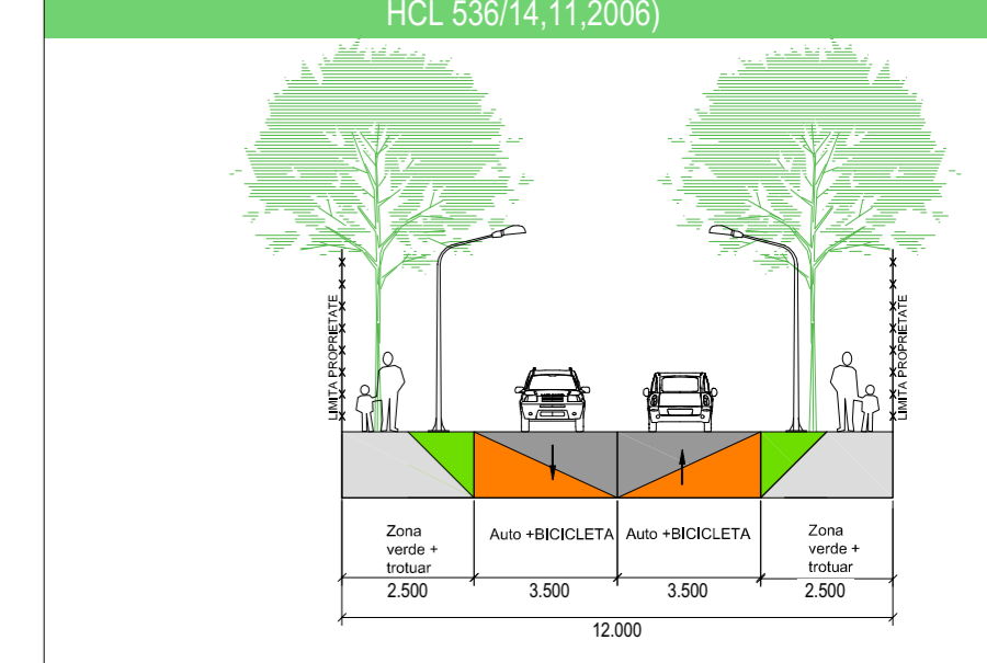
Profil transversal propus de specialist drumuri - latime 12m, (conform PUZ Cnstr. industriale-depozitare si servicii, aprobat prin HCL 536/14,11,2006)
