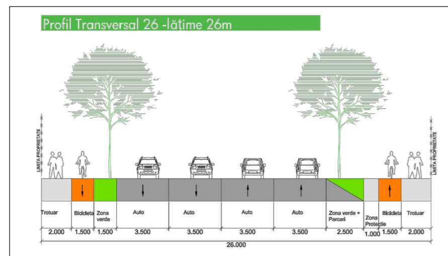
Profil transversal PT 26 - conform PUG Etapa 3
