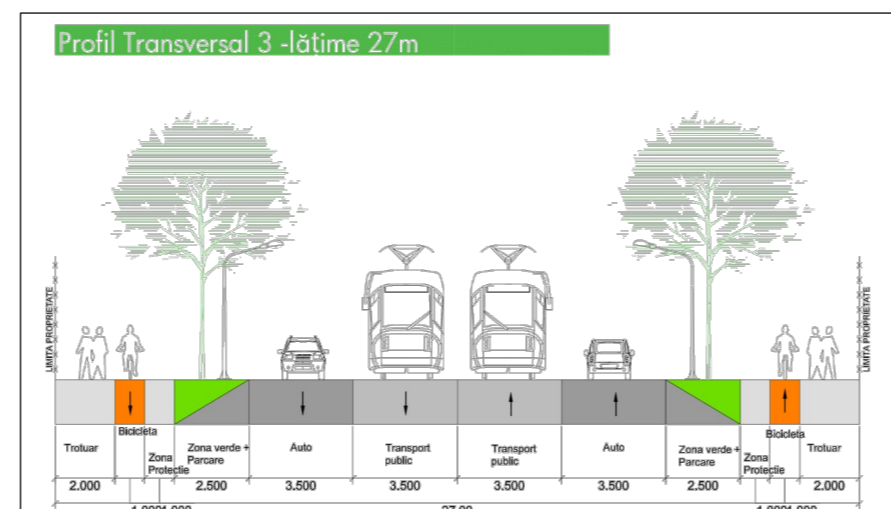
Profil transversal PT 3 - conform PUG Etapa 3
