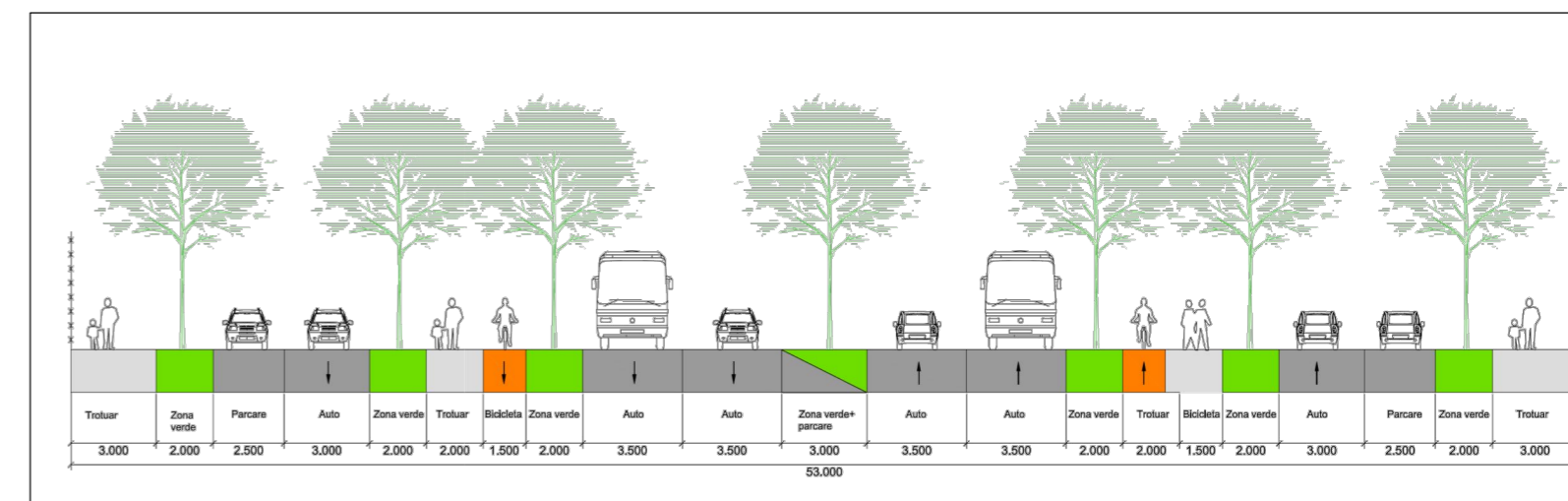
Profil transversal PT 23 (53m) - conform PUG Etapa 3
