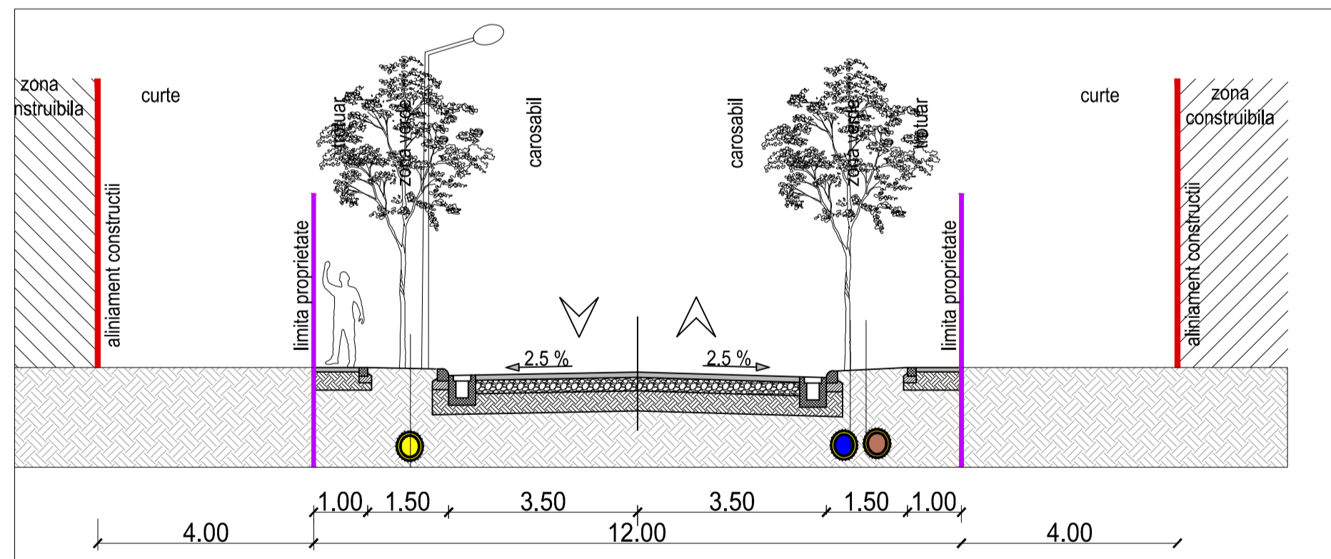
PROFIL STRADAL TRANSVERSAL - STRADA BISTREI - 12.00 m Scara 1:100
