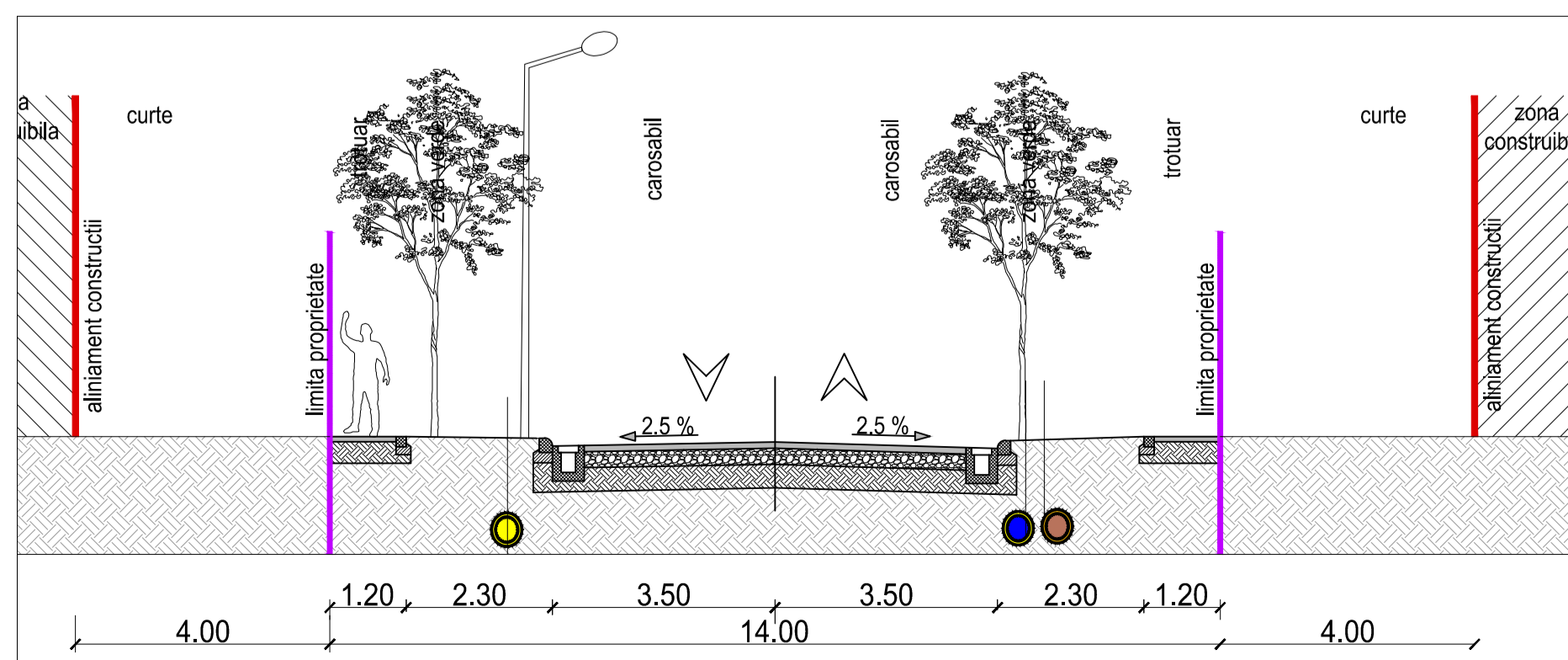
PROFIL STRADAL TRANSVERSAL - CALEA MOSNITEI - 14.00 m Scara 1:100
