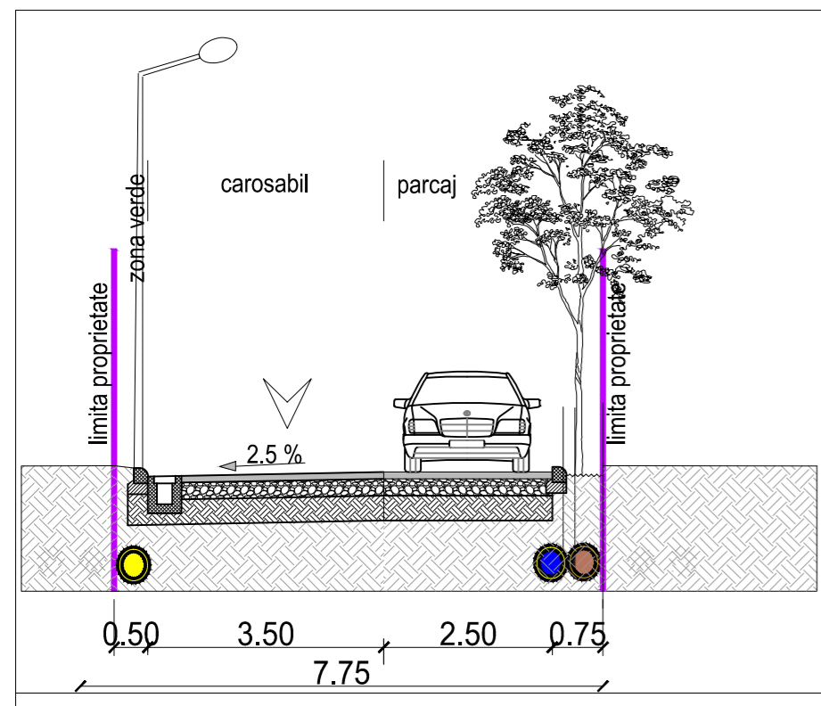
PROFIL TRANSVERSAL - SUPRAFATA CAROSABILA PE PARCELA Scara 1:100
