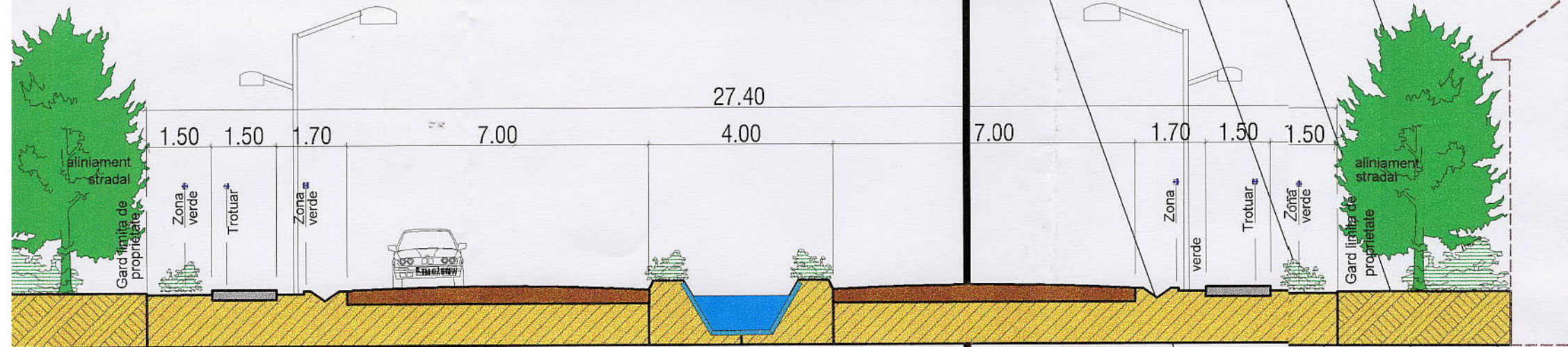
PROFIL TRANSVERSAL STRAZI NOI SECUNDARE sectiunea A
