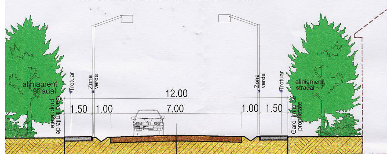
PROFIL TRANSVERSAL STRAZI NOI SECUNDARE sectiunea A
