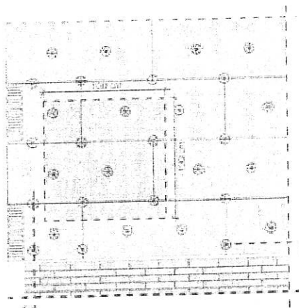
Dispunerea diblurilor pentru fixarea plăcilor din vată minerală bazaltică (MVB) în zona colțului la colțul în câmp curent
