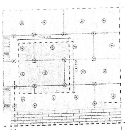
Dispunerea diblurilor pentru fixarea plăcilor din vată minerală bazaltică (W) în zona nodului la cel și în câmp curent.
