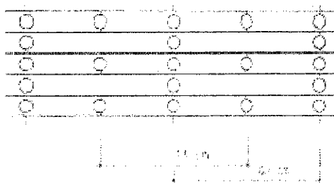
Dispunerea diblurilor pentru fixarea plăcilor din vată minerală bazaltică (MW) în zona soclului, la colț și în câmp curent.
