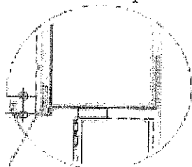
Plasa se poartă 1 cm peste profilul de beton
