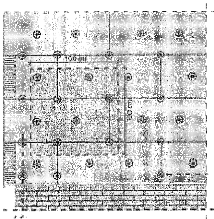
Dispunerea diblurilor pentru fixarea plăcilor din vată minerală bazaltică (MW) în zona colțului la colț și în câmp curent.
