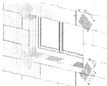
Armarea suplimentară a colțurilor
