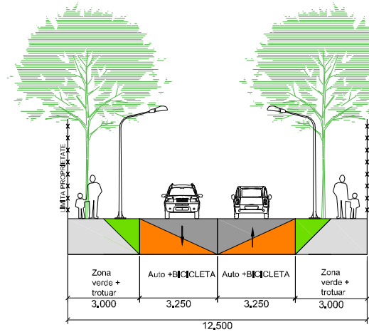
Profil Transversal 47 -lățime 12.5m
