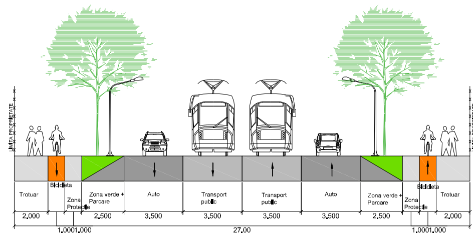
Profil Transversal 70 -lățime 24m
