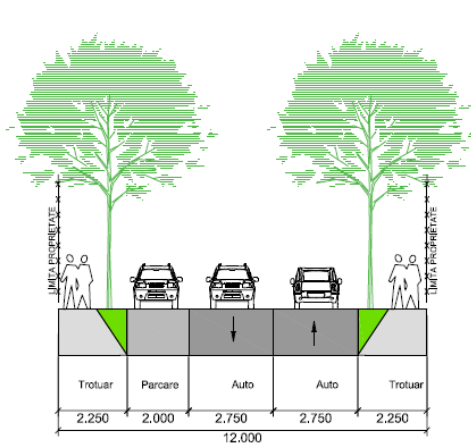
Profil Transversal 40 -lățime 12m
